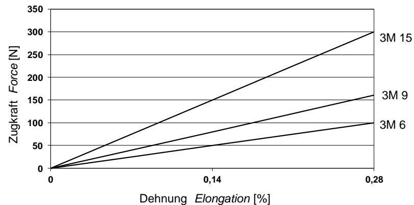
Dehnung Elongation
