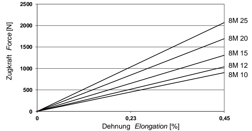
Dehnung Elongation
